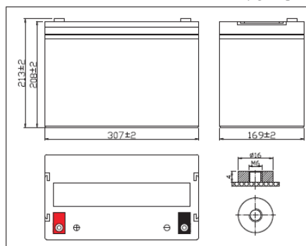
Клеммы T1
