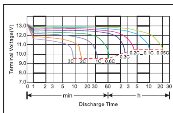
Разрядный ток 25°C
